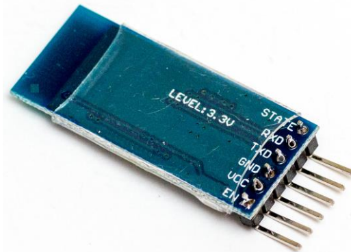
Figura 1. Descripción de los pines del Bluetooth Comercial HC-05.
